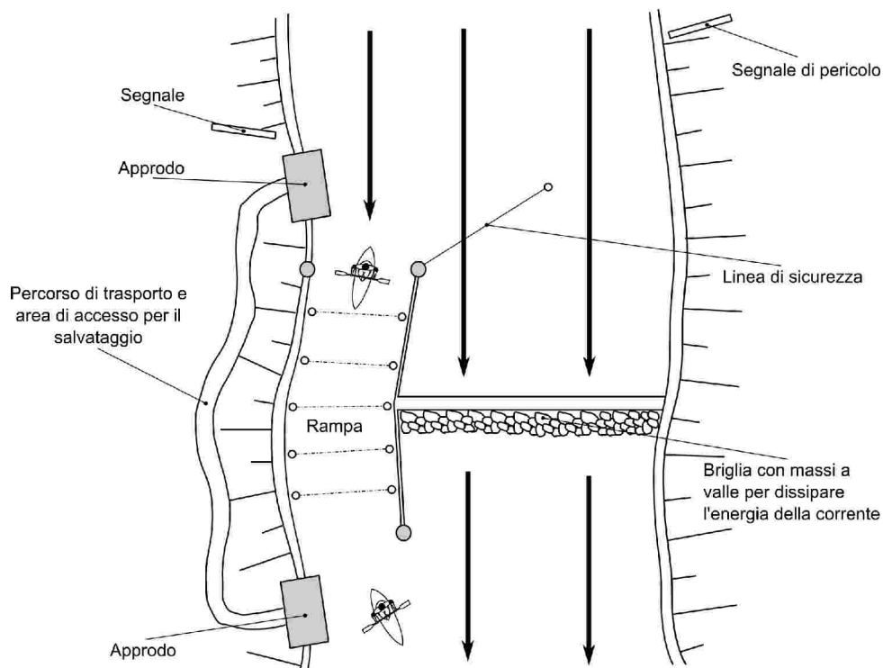
Figura 6.7: schema di una rampa per canoe con approdi per il trasbordo (disegno modificato tratto da Schwarz, 1993).
