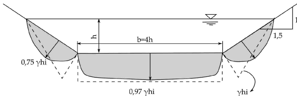
Figura A.9: distribuzione reale delle tensioni in un alveo trapezoidale (modificato da Lane e Carlson, 1953). La linea tratteggiata rappresenta i valori che si avrebbero nel caso si applicasse la sola relazione \gamma h i , con h decrescente sulla sponda.
