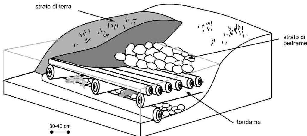
Figura 5.4: schema di un rifugio per pesci tipo realizzato con tondele.
