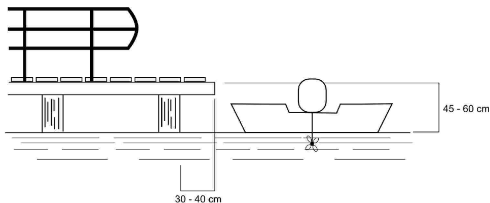
Figura 6.10: schema di un pontile fisso (disegno modificato tratto da Toccolini et al., 2004).
