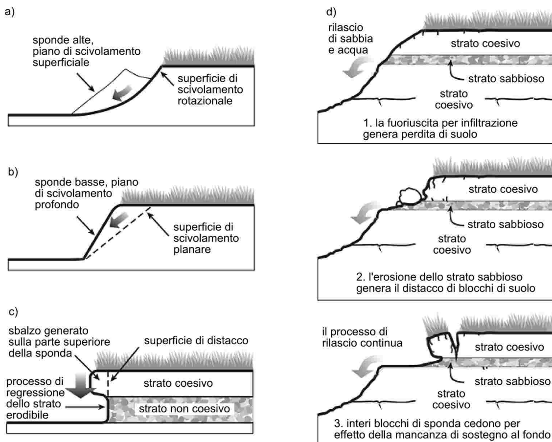
Figura A.13: tipologie di instabilità di sponda a) fenomeni rotazionali, b) fenomeni planari, c) crolli, d) sifonamenti.
