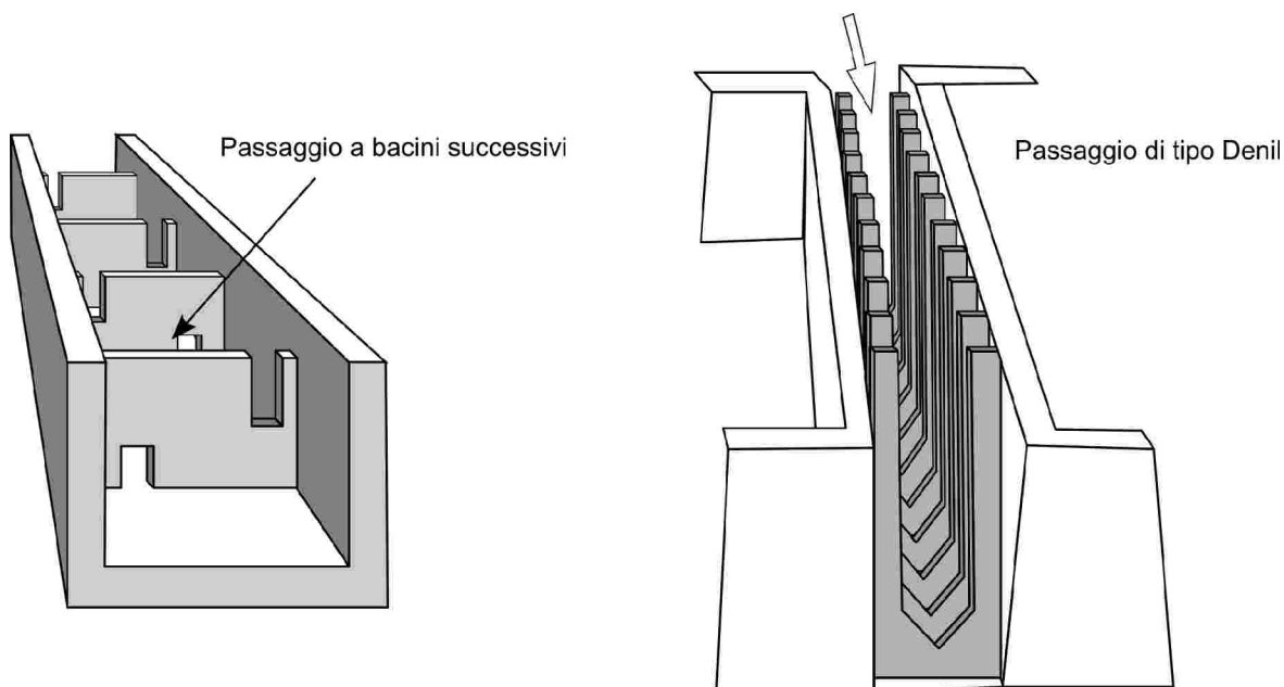
Figura 5.8: passaggi per pesci “a bacini successivi” e di tipo Denil (ridisegnato da Loro e Zabetti, 1990).
