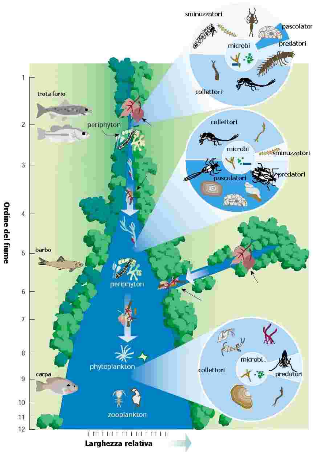
Figura 2.13: relazioni proposte dal River Continuum Concept tra le dimensioni del corso d'acqua ed i graduali aggiustamenti nella struttura e nelle funzioni delle comunità lotiche (da FISRW, 2001).
