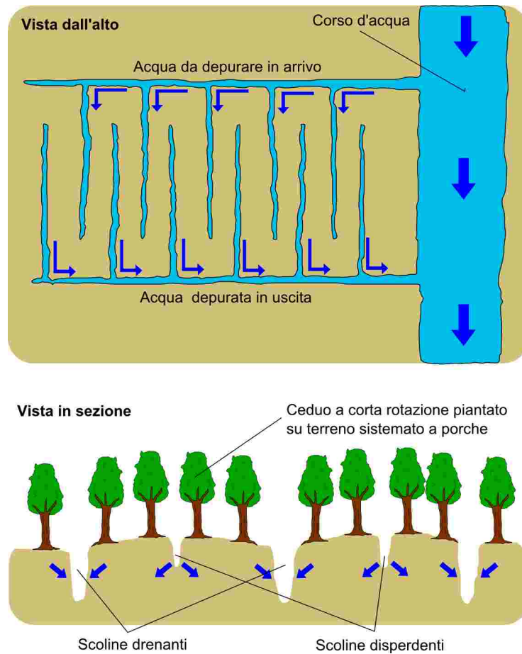
Figura 5.18: schema di ceduo a corta rotazione con funzione depurativa. Dal reticolo delle scoline disperdenti l'acqua da depurare prelevata dal corso d'acqua si infiltra nel terreno ed entra in contatto con gli apparati radicali degli alberi della SRF, che depurano l'acqua fisicamente e biologicamente. Il reticolo delle scoline drenanti, più profonde a causa della sistemazione a baulature (o a porche) del terreno, cattura l'acqua depurata e la restituisce al corso d'acqua (disegno modificato di Giovanni Trebbiani, da Mezzalira, 2005b).
